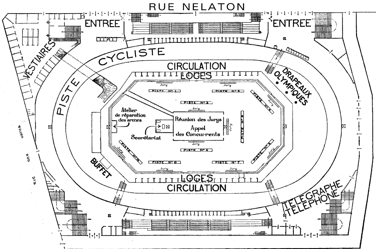
PLAN DU VÉLODROME D'HIVER AMÉNAGÉ PAR LE C. O. F. POUR LES ÉLIMINATOIRES DES ÉPREUVES DE FLEURET.
